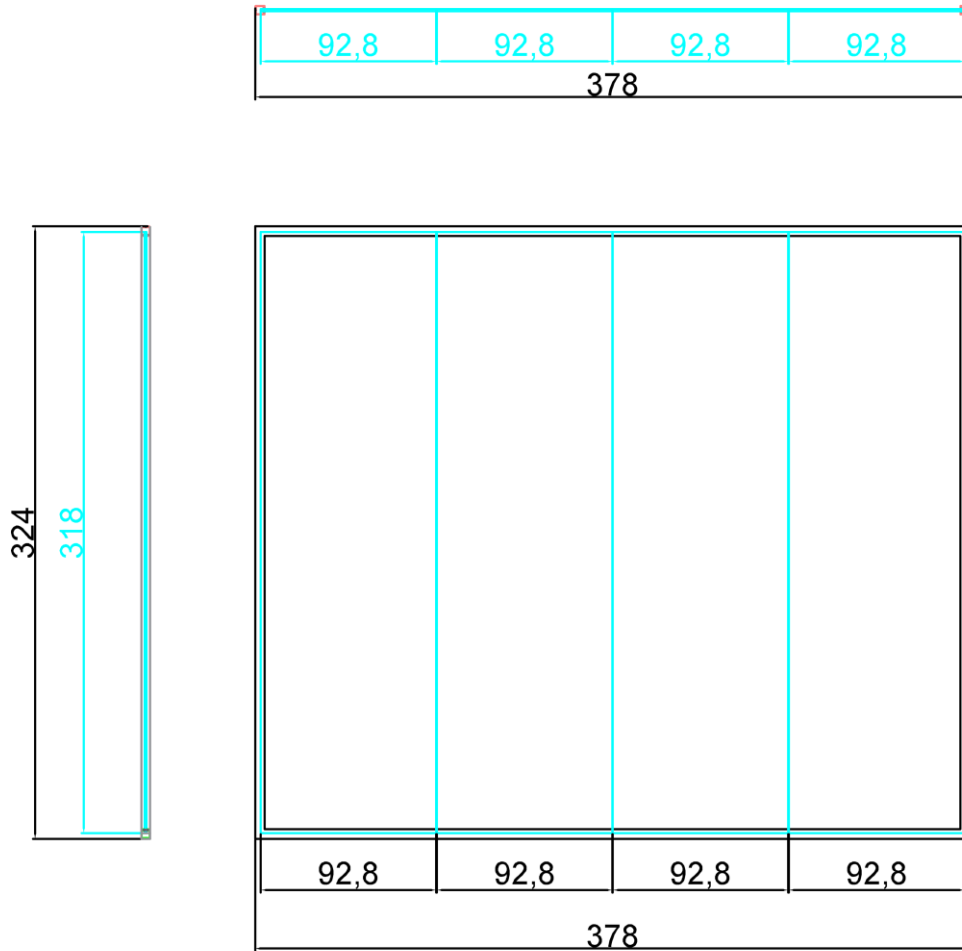
Şekil 3.1 Teknik Çizim 1
