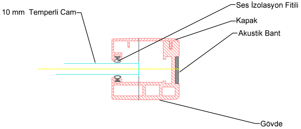
Şekil 3.2 Teknik Çizim 2
