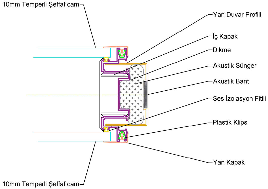
Şekil 3.2 Teknik Çizim 2
