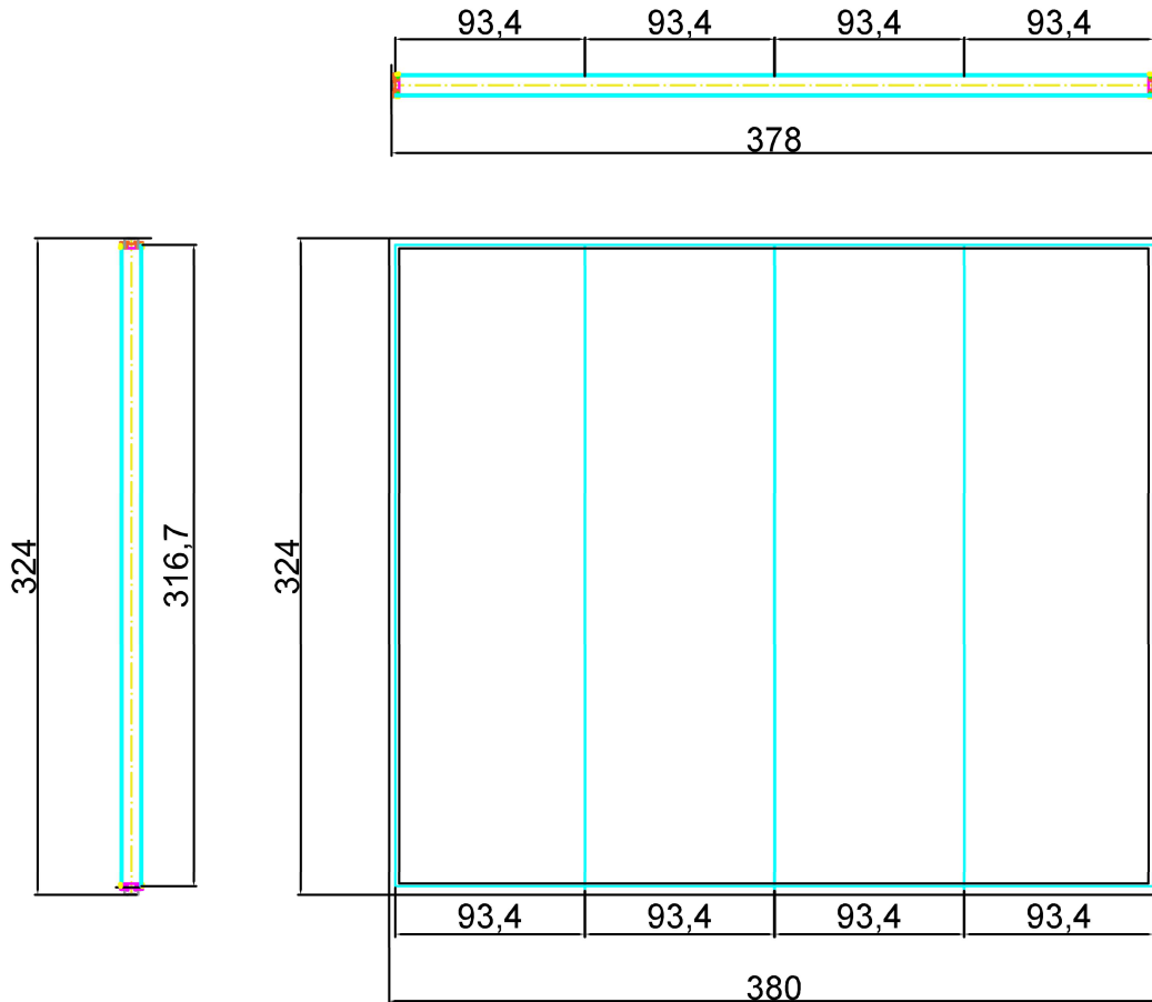
Şekil 3.1 Teknik Çizim 1
