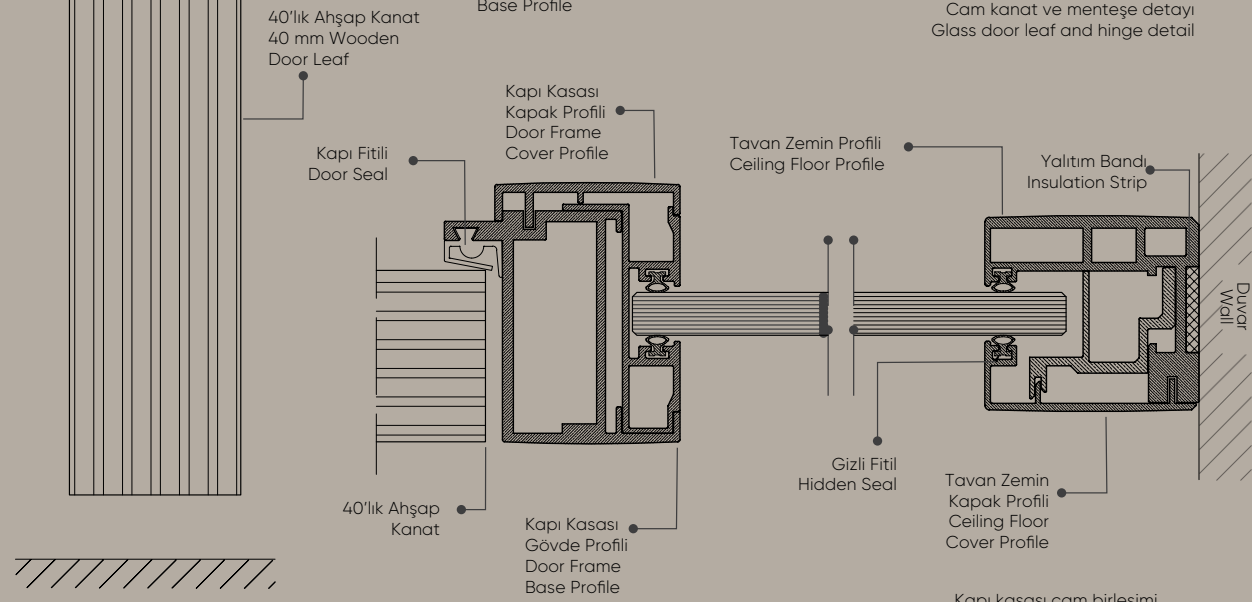
Kası kasası düşey kesit (Ahşap kanat) Door frame vertical section (Wooden door leaf)
